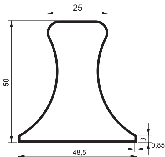
TG-022 Peso: 0,508kg/m Embalagem: 6 un. Régua bitubular
