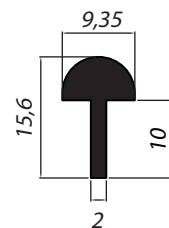
TPE001 Peso: 0,191 kg/m Trilho de embutir/trilho macarrão
