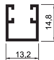
BG-007 Peso: 0,170kg/m Embalagem: 5 un. Perfil U com escova
