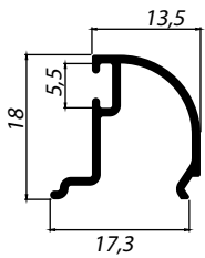
ILG026 Peso: 0,165 kg/m
