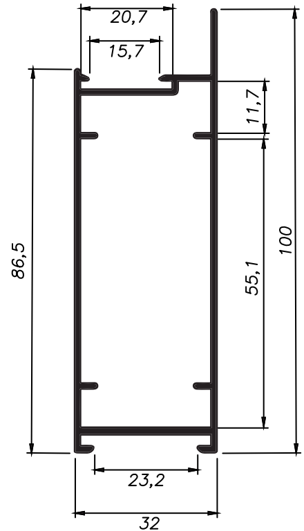
ILG042 Peso: 1,035 kg/m Embalagem Especial
