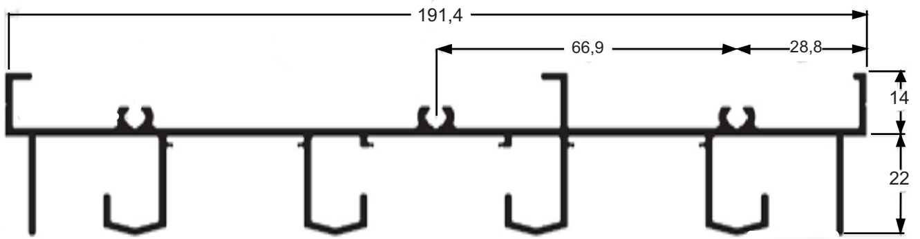
TLG070 Peso: 2,273 kg/m
