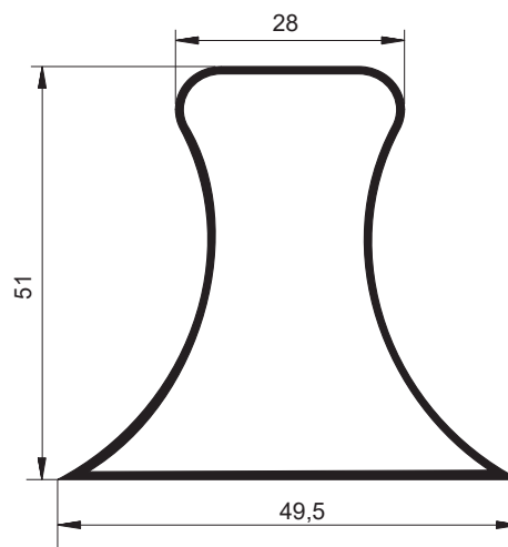
TG-021 Peso: 0,421kg/m Embalagem: 5 un. Régua tubular com "pega"
