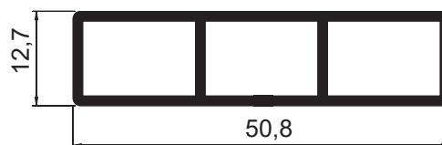
MV-053 Peso: 0,555kg/m Embalagem: 10 un. Tubo retangular tritubular com raio
