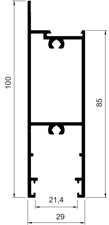
ILG007 Peso: 1,211 kg/m Embalagem Especial
