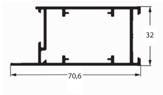
TLG083 Peso: 0,410 kg/m
