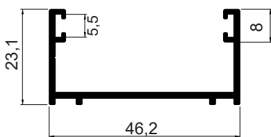
ILG028 Peso: 0,445 kg/m
