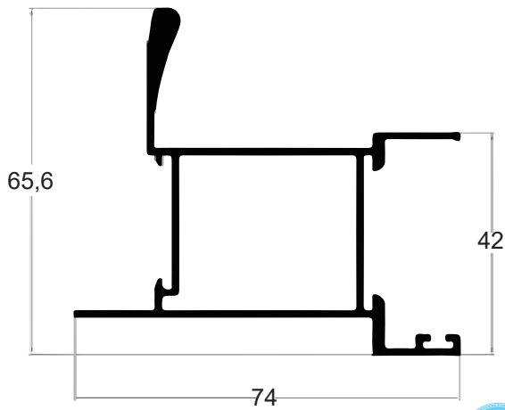
TLG020 Peso: 1,116 kg/m Embalagem Especial
