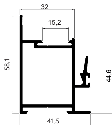
ILG049 Peso: 0,923 kg/m
