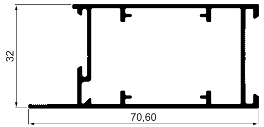
ILG043 Peso: 0,856 kg/m
