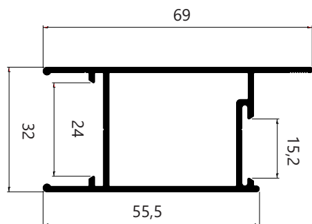
ILG050 Peso: 0,781 kg/m
