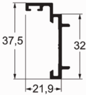
TLG016 Peso: 0,338 kg/m
