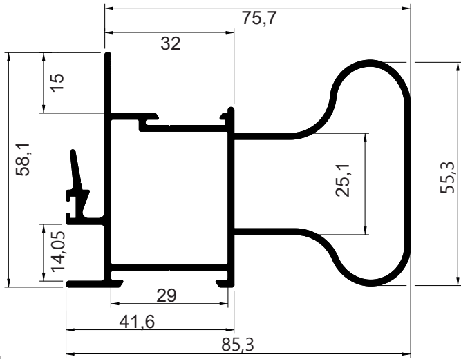
ILG021 Peso: 1,558 kg/m Embalagem Especial
