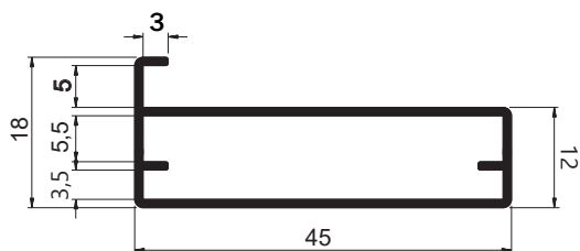
MV-067 Peso: 0,351kg/m Embalagem: 8 un. Moldura para vidro 5mm
