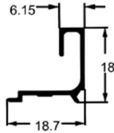
TLG027 Peso: 0,149 kg/m
