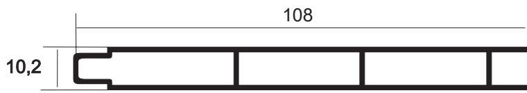
LB-005 Peso: 0,769kg/m Embalagem Especial: 4 un. Lambri tubular reto
