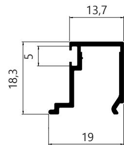
IBG057 Peso: 0,178 kg/m
