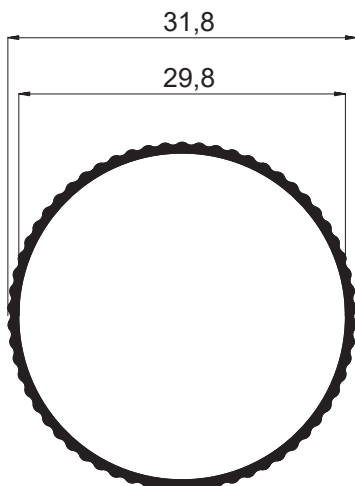
DS-072 Peso: 0,240kg/m Embalagem: 6 un. Tubo redondo estriado 31,8mm
