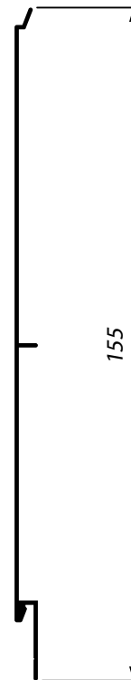
TFP001 Peso: 0,252kg/m Embalagem Friso de porta Cromado p/ Lambri - Barra 3 metros
