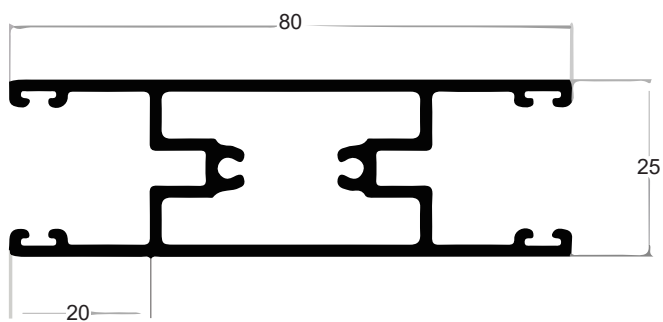
IMN007 Peso: 0,677 kg/m
