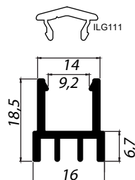
ILG157 Peso: 0,255 kg/m
