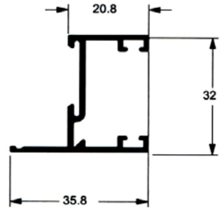
TLG083 Peso: 0,410 kg/m
