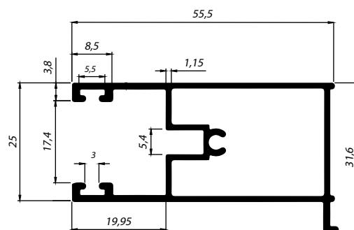
IMN007 Peso: 0,677 kg/m
