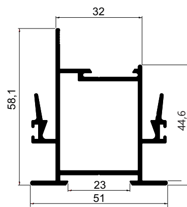
ILG162 Peso: 1,109 kg/m
